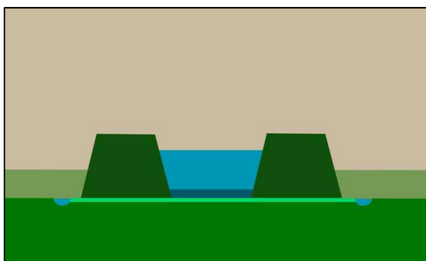
De Selwerder grondzijl onder het Westerdiep
