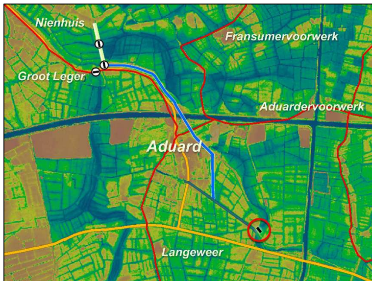
Reconstructie van het tracé van het kanaal naar de zijl bij de Arbere met de veronderstelde dam in de Kliefslootgeul (in de cirkel)
