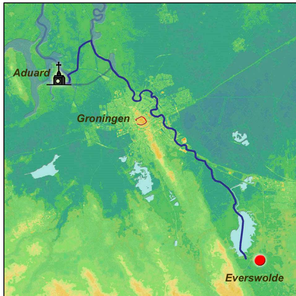
Een nieuwe verbinding tussen de Hunze en Aduard; eind 13 e eeuw (?)
