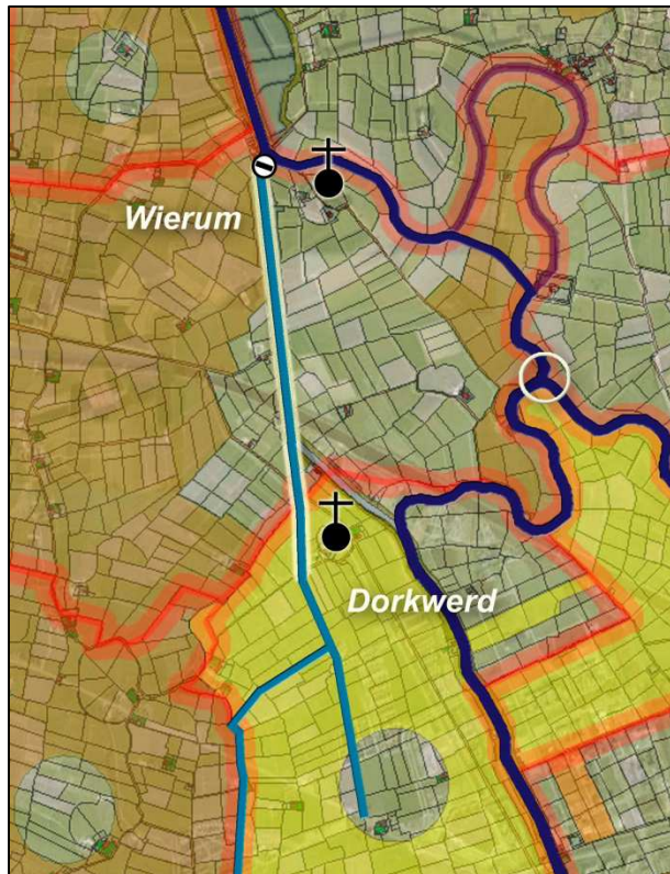
Een nieuwe zijl bij Wierum (c. 1360)
