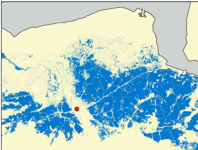
Het 'winterwater' volgens H. Dijkema (1851) 1
