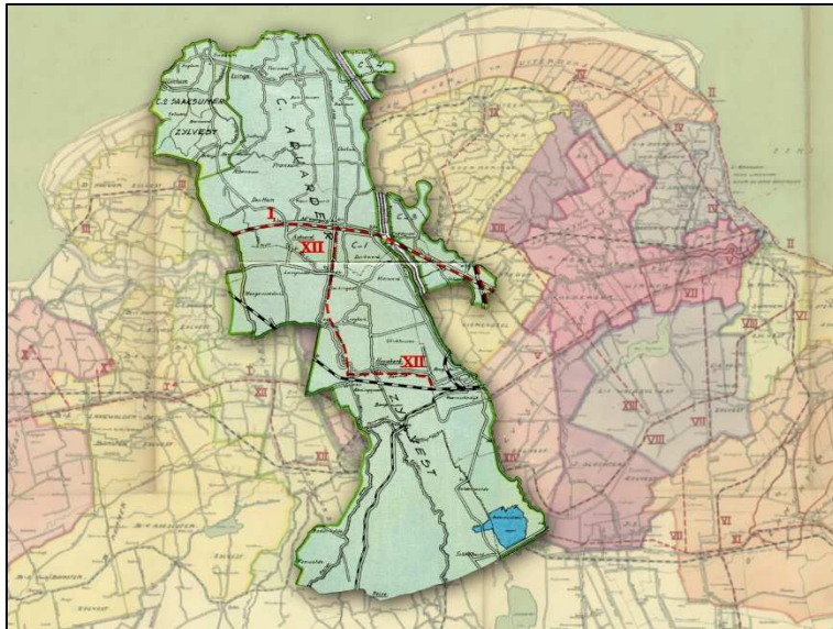
Het Aduarderzijlvest naar J. Kooper (1939)
