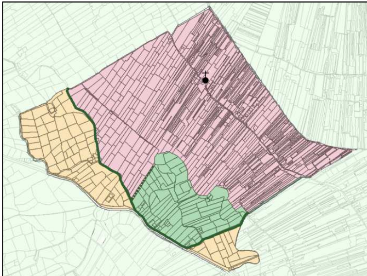
De verkavelingspatronen in Engelbert
