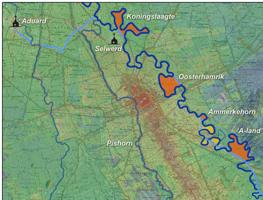
Vroege bochtsafsnijdingen tussen Westerbroek en Paddepoel
