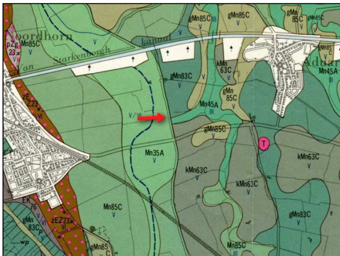
Grondsoorten tussen Zuidhorn en Aduard
