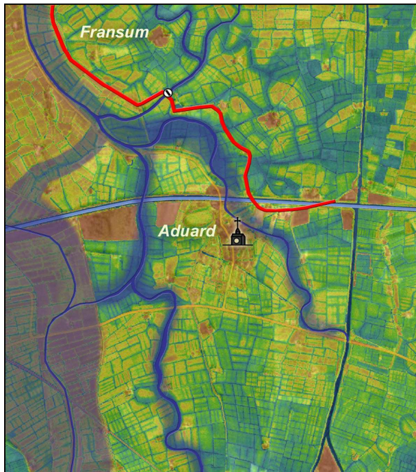
Middagsterdijk met sluis
