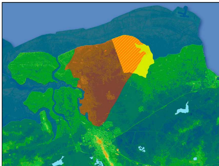
Winsumer- en Oosterniezijlvest Roodachtig: het oude Winsumerzijlvest Geel: het zuidelijke deel van het Oosterniezijlvest Rood-geel gestreept: het in het Winsumerzijlvest ingelaten noordelijke deel van het Oosterniezijlvest
