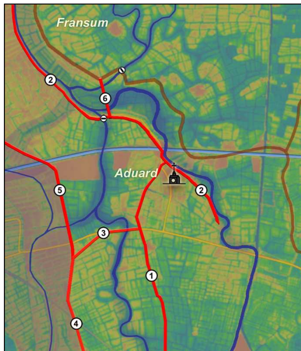
Enkele vroege ingrepen op één plaatje
