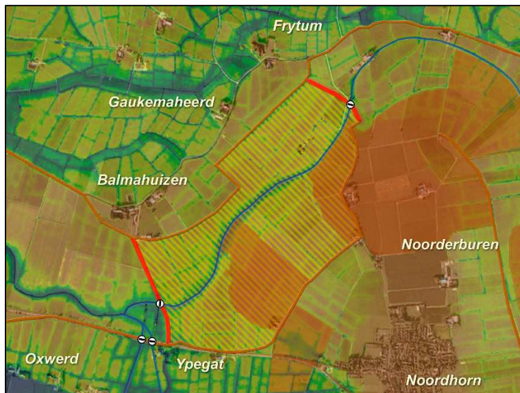
De uiterdijkslanden tussen Balmahuizen en Noorderhorn
