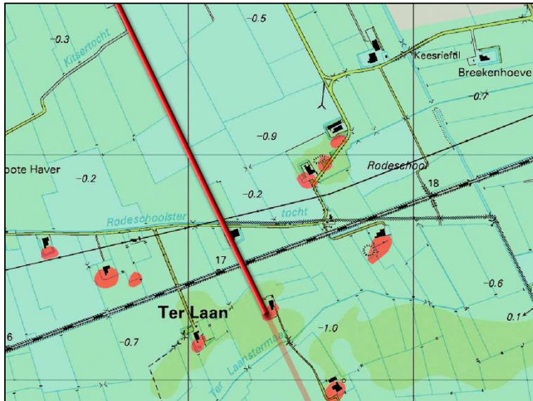
Rodeschool en de raailijn op Warffum
