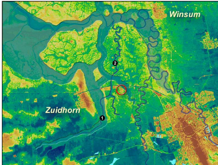
Inbraakgeulen en oude rivieren
