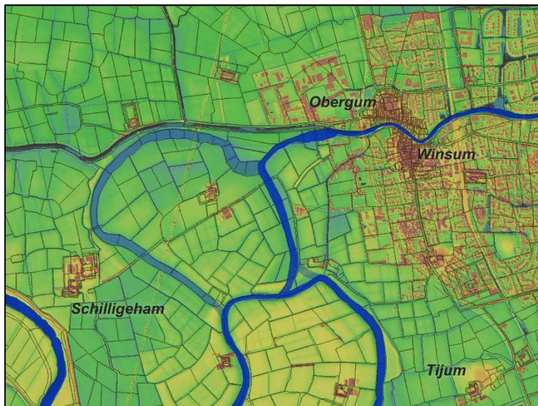
De 'Baatjeborg-kronkel' afgesneden: 'monnikenwerk'?
