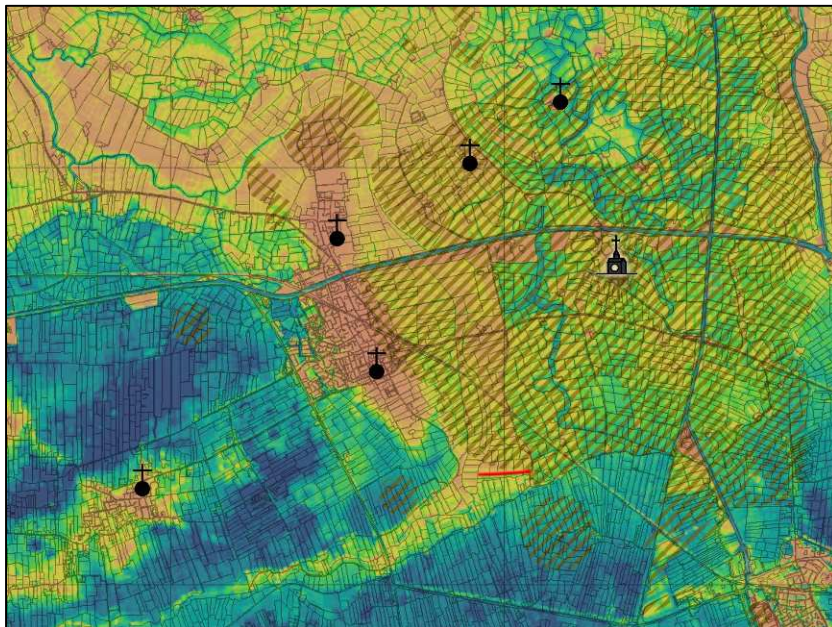
Aduard en de 'Woldgeul'
