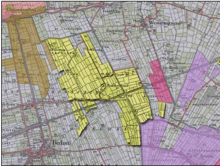
Het Aduarderland bij Rodeschool
