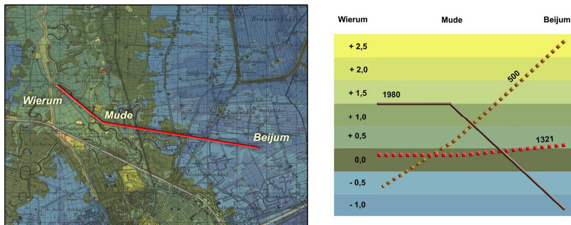
Schematische voorstelling van de bodemdaling in het Woldland
