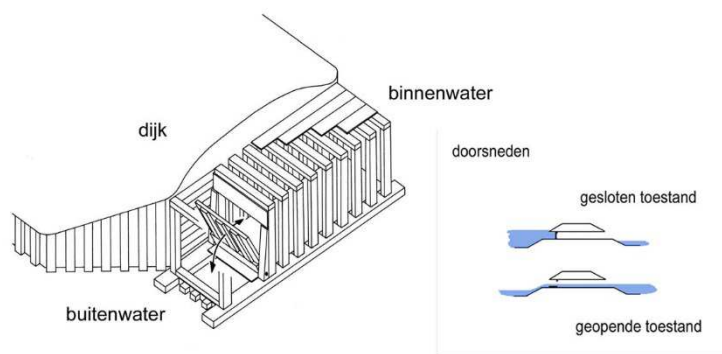
Reconstructietekening van een dertiende-eeuwse pomp
